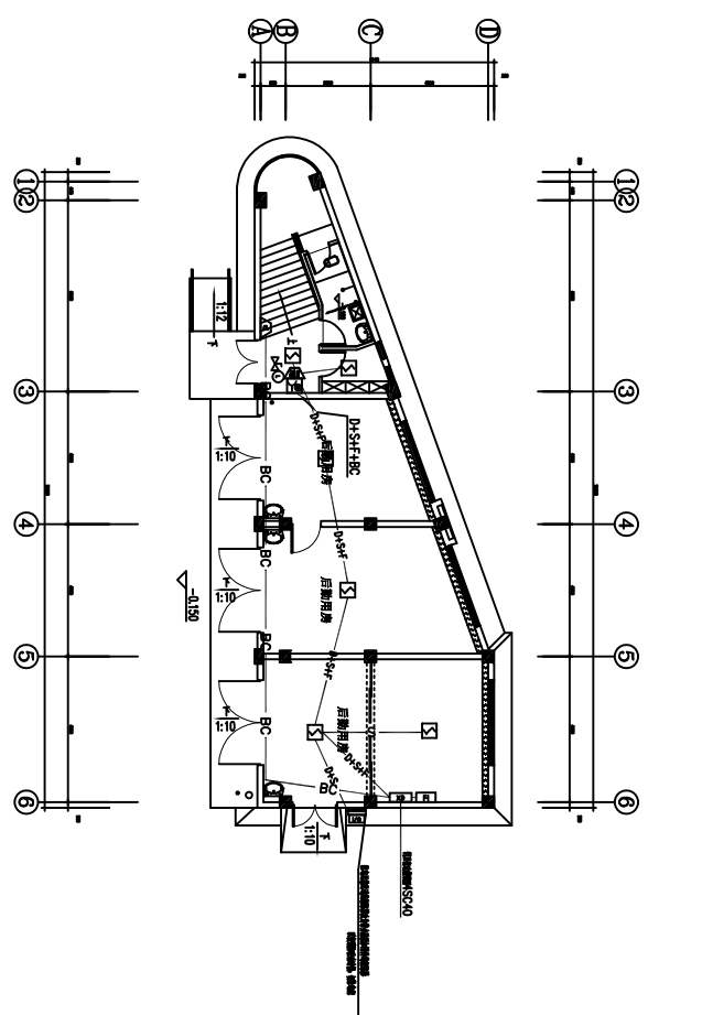
一层大会议室平面图 1:100
